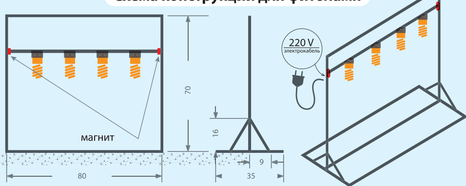
Схема конструкции для фитоламп
